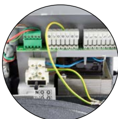
PROGRAMMATORE ELETTRONICO CON MORSETTIERE ETRAIBILI
